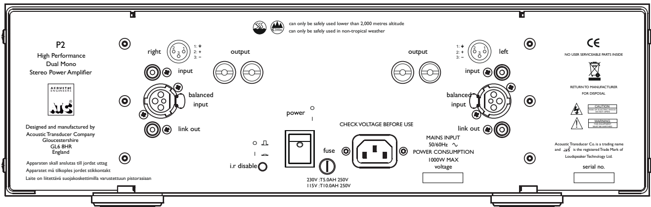
Diagramm 3 - P2 Rückwand und Anschlussbuchsen
