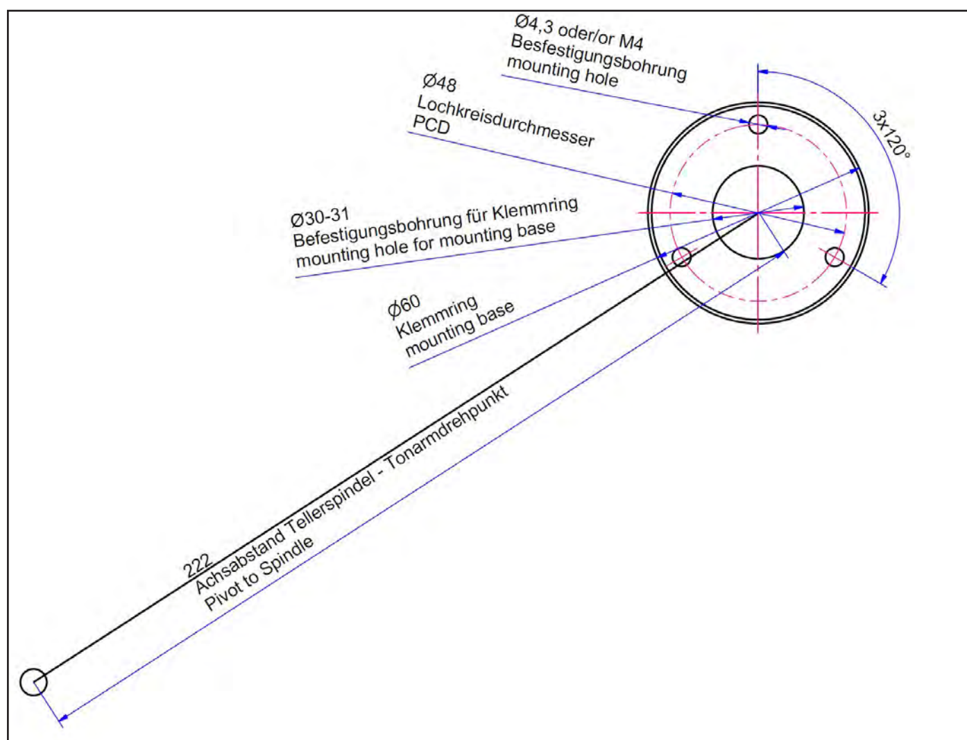
Abb. 3: Bohrschablone für die Montage des Klemmrings auf einem Laufwerk eines anderen Herstellers
