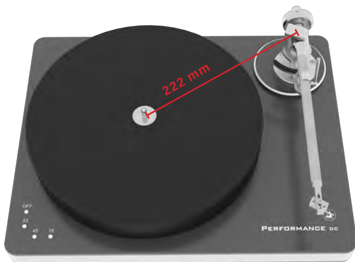
Abb. 7: Abstand der Spindel zum Drehpunkt des Tonarms
