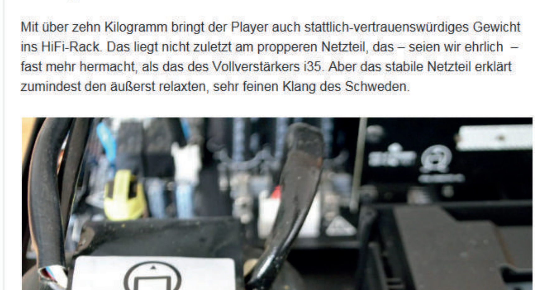
Erstaunlich kräftig: der Träfo des CD35 ist größer als der des Vollverstärkers i35 und sorgt für jederzeit ausreichende Spannungsverhältnisse (Foto: H. Biermann)
