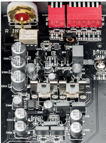
Direkt an den Eingangsbuchsen sitzen die DIP-Schalter für die präzise Anpassung an den verwendeten Tonabnehmer
