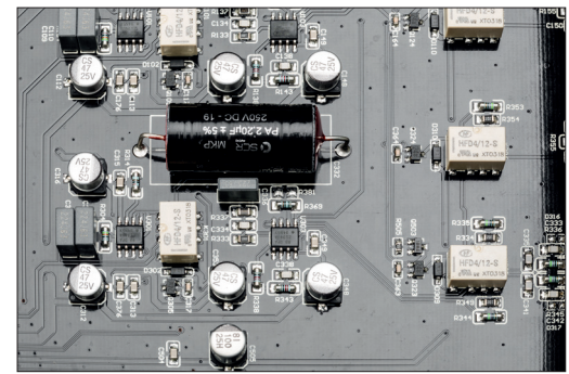
Ausnahmsweise nicht in SMD-Technik findet sich in der Ausgangsstufe ein hochwertiger Folienkondensator
