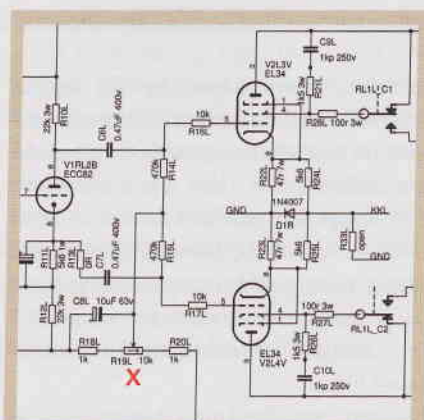
GEMEINSAMER AUFTRIFF: Das Justage-Potentiometer (X) stellt den Ruhestrom für beide Gegentakt-Endröhren gleichzeitig ein.
